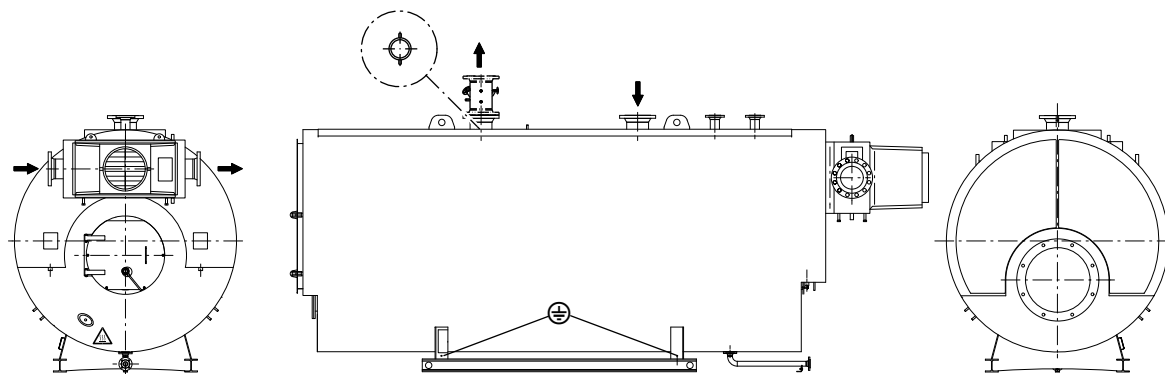
Рис. 14 Неконденсационный экономайзер
