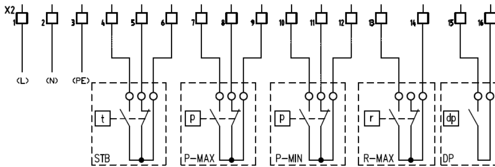
Рис. 2 Схема подключения внешних устройств колодка X2
