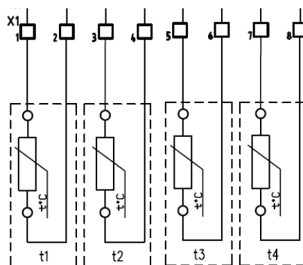
Рис. 4 Схема подключения внешних устройств колодка X1
