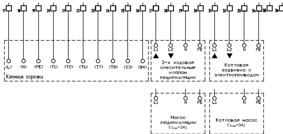
Рис. 3 Схема подключения внешних устройств колодка X2 продолжение
