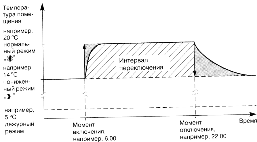
Пример установленной на заводе программы выдержек времени
