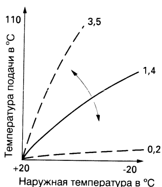
Изменение крутизны отопительной характеристики
