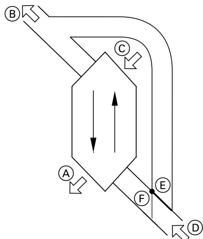
Рис. 70 Пример: Vitovent 300-F
