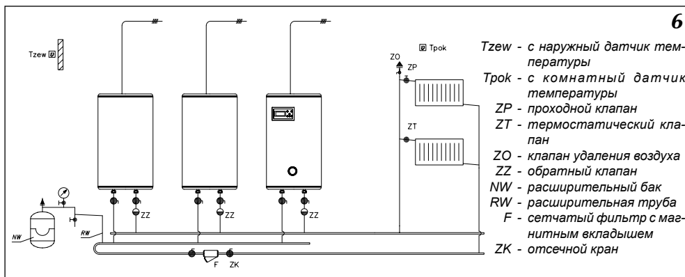
Рис.6 Подключение группы котлов.
