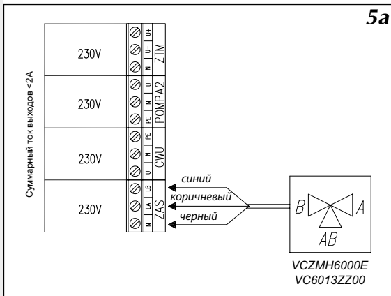
Рис.5а Схема подключения клапана Honeywell
