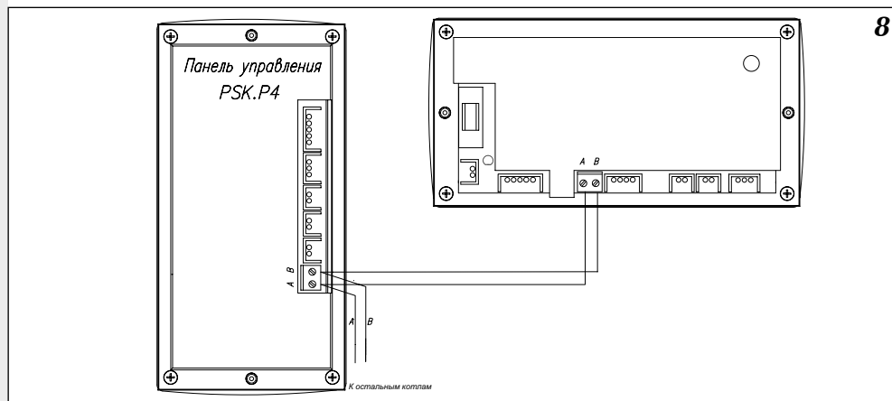
Рис.8 Подключение панелей управления группы котлов
